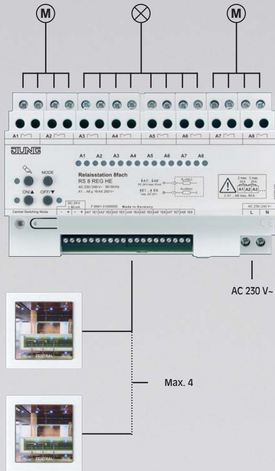
Beispielanschluss Sensormodul Example for sensor module connection
